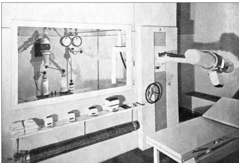
Aparato de Radioterapia «Stavilivolt». Número extraordinario del Boletín de Alumnos Internos. Junio, 1936.
